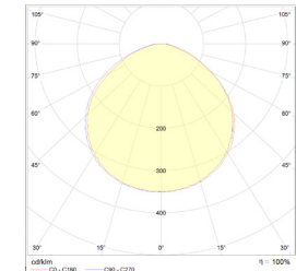
KRZYWA ROZSYŁU 110° DISTRIBUTION CURVE 110°
