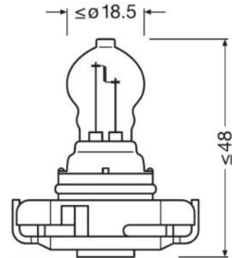
PSX24W
